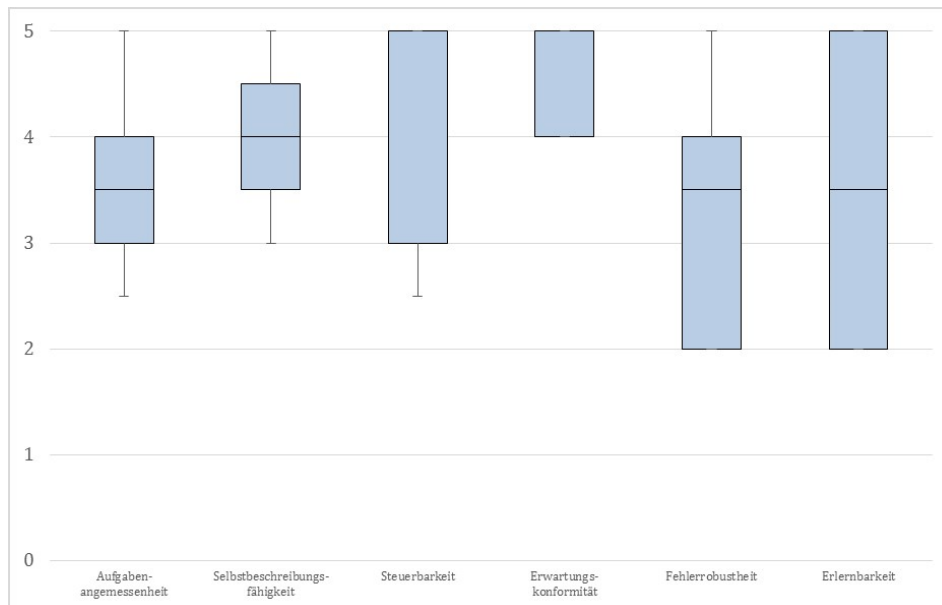
Abbildung 3: Ergebnisse der Usability-Prüfung der Anwendung „elektronische Überleitung“ auf Basis des HL7 CDA Standards ePflegerbericht (n=7)
